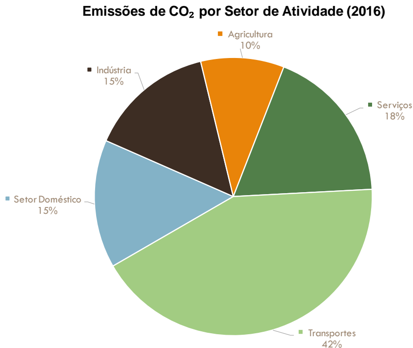
Figura 52 - Emissões de CO 2 por Setor de Atividade em 2016 [%]
