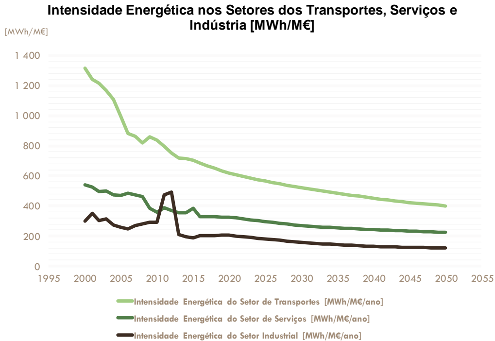
Figura 22 - Intensidade Energética nos Setores Transportes, Serviços e Indústria [MWh/M€/ano]
