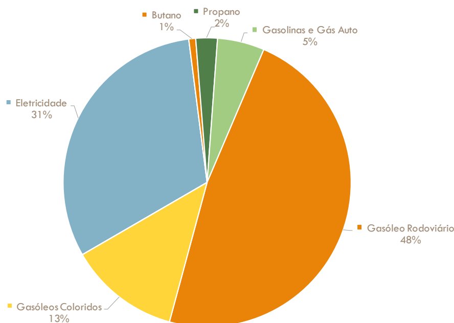
Emissões de CO 2 por Vetor Energético Consumido (2016)
